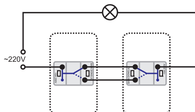
Схема 2. Подключение 2-х переключателей для включения нагрузки с двух мест
