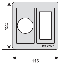
размеры двухместных рамок WST 2036 (1-я Розетка + TV)
