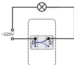
Схема 1. Подключение переключателя для включения нагрузки с одного места (как обычный выключатель)
