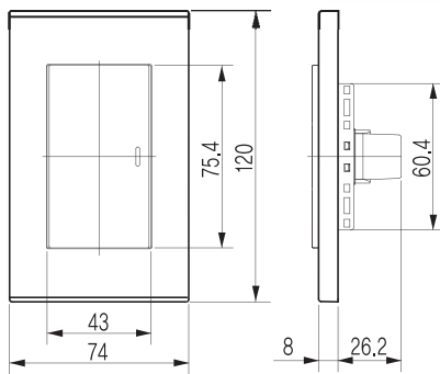
WRC 2421 Переключатель 1-клавишный Матовое серебро
