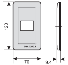
размеры одноместных рамок WST 1921 (рамка TF.1)
