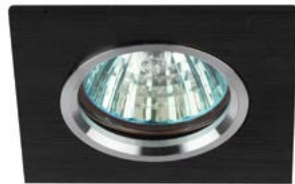
KL57 SL-BK серебро/черный ↔ 120x120мм 105 мм ↓ 20 мм → 220V
