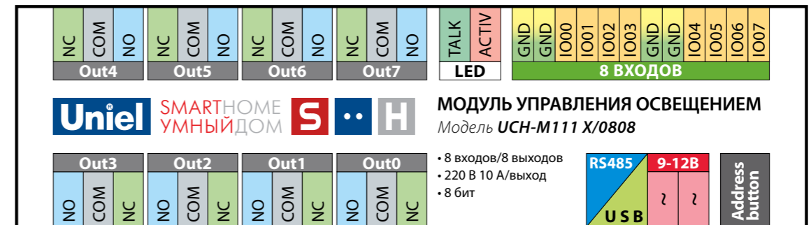
ВЫХОДЫ УПРАВЛЯЮЩИХ РЕЛЕ ДЛЯ ПОДКЛЮЧЕНИЯ ИСТОЧНИКОВ СВЕТА
