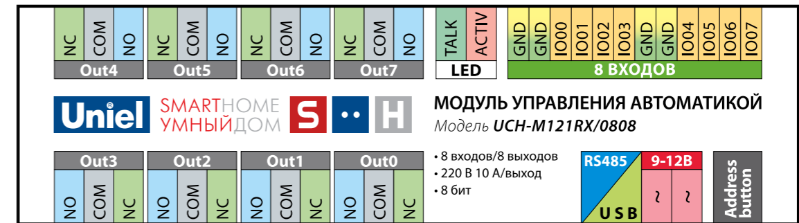
ВЫХОДЫ УПРАВЛЯЮЩИХ РЕЛЕ ДЛЯ ПОДКЛЮЧЕНИЯ ЭЛЕКТРОПРИБОРОВ
